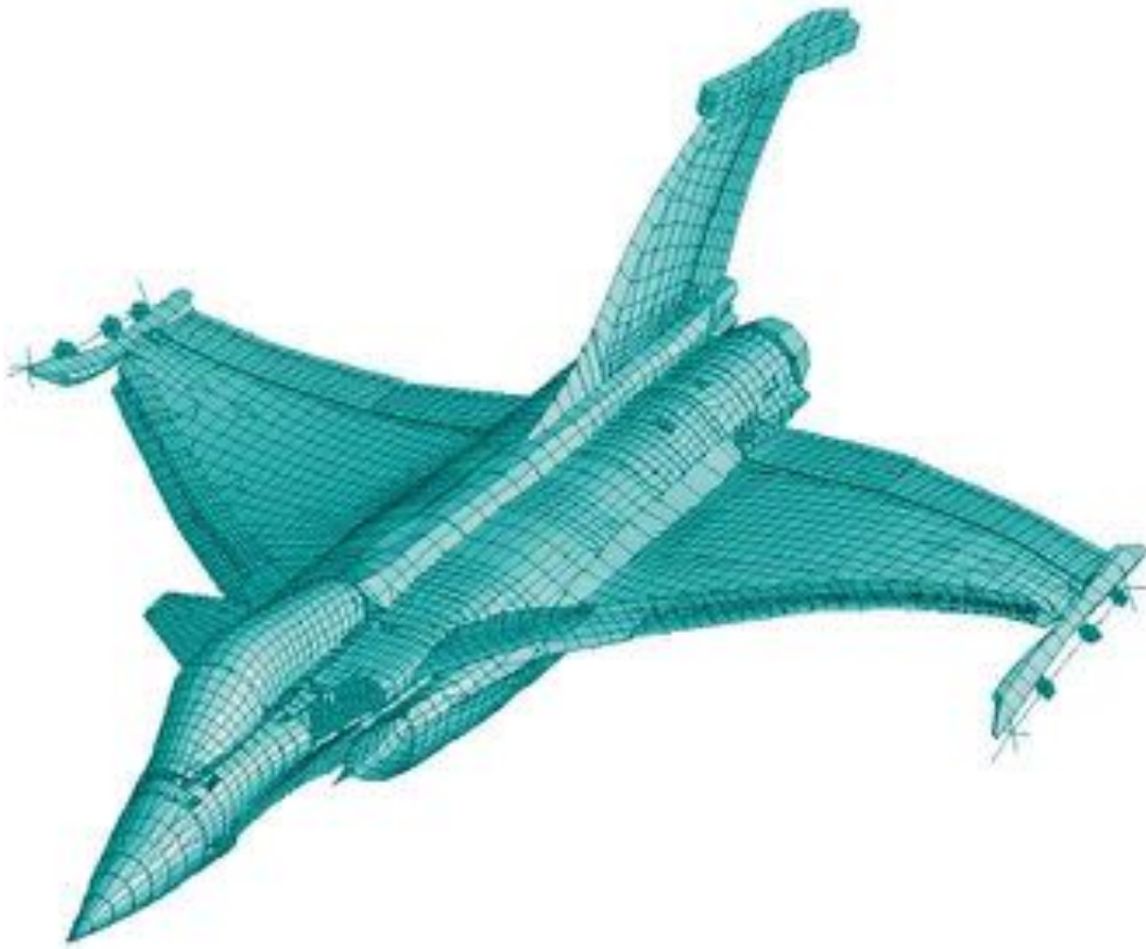
Fig. 21 Les calculs par éléments finis permettent une très bonne prédiction des modes de vibration : ici premier mode antisymétrique du Rafale, calcul Dassault Aviation
