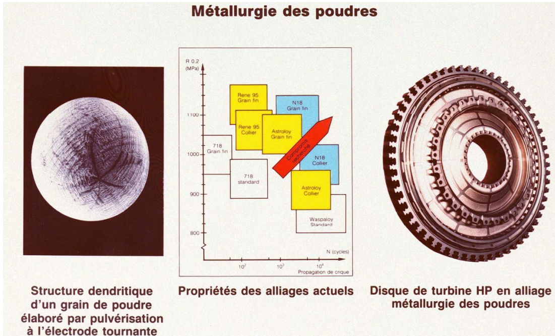
Fig. 51 Métallurgie des poudres et alliage N18
