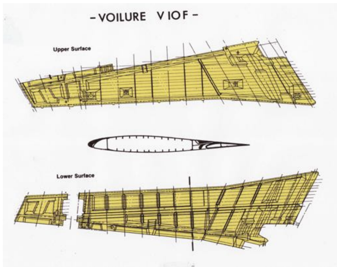
Fig. 44 V 10 F dessin du caisson de voilure en composite
