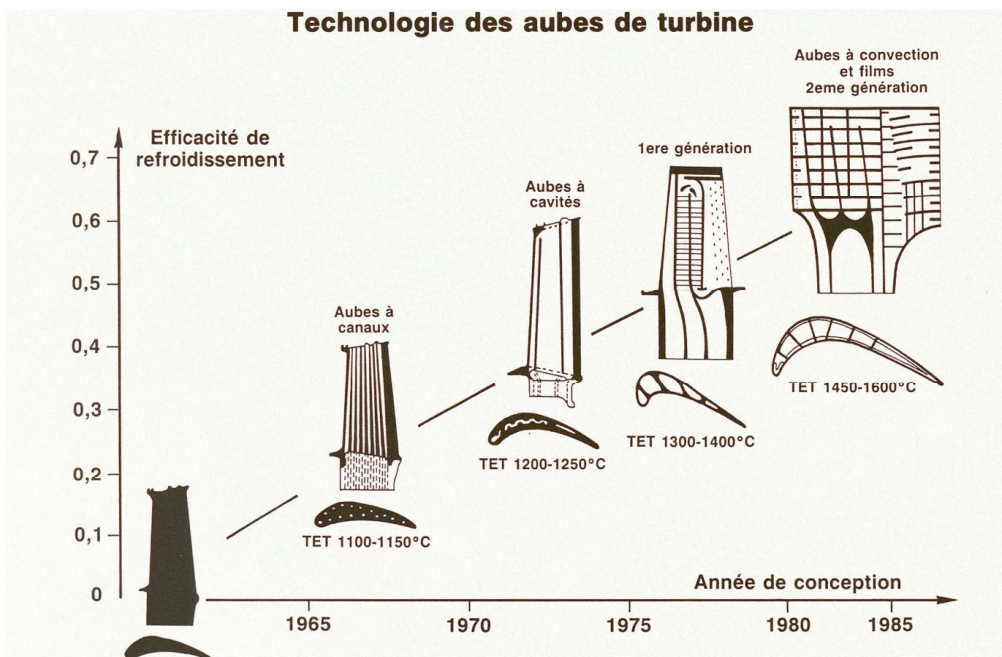
Fig. 30 Technologie des aubes de turbines refroidies (Source SNECMA)
